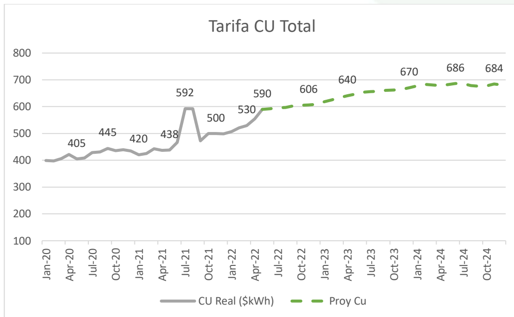
Fig 10. Proyección tarifa cargos totales (construcción propia)
