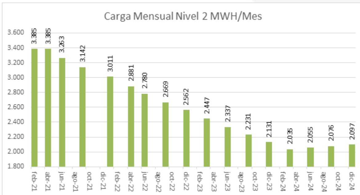
Fig 11. Proyección de la demanda del sistema (construcción propia – SIAP)
